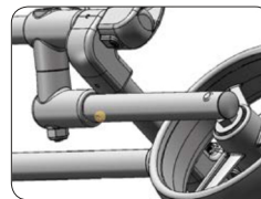
Vorderrad - Geradeauslauf Trolley läuft nach links: Schraube im Uhrzeigersinn drehen. Trolley läuft nach rechts: Schraube gegen den Uhrzeigersinn drehen.
